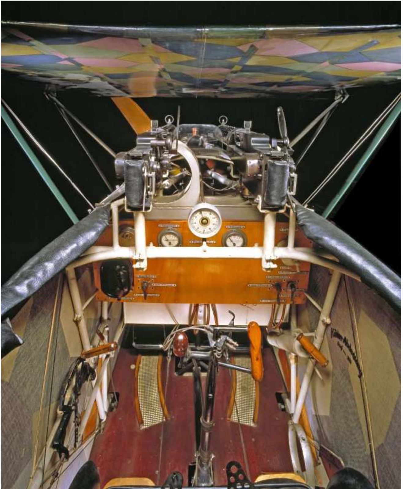
Fokker D.VII
